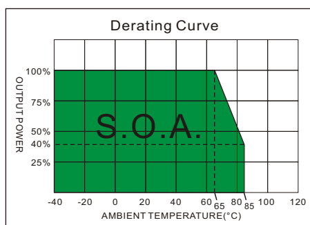
MR-7812-0.5
