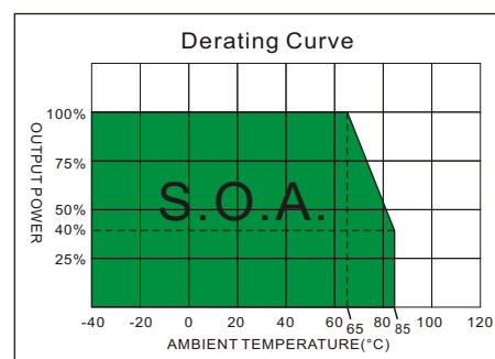
MR-7815-0.5
