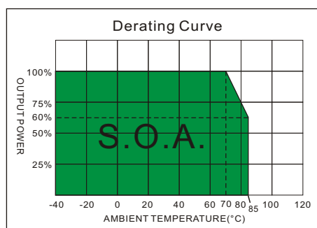
MR-7805-0.5
